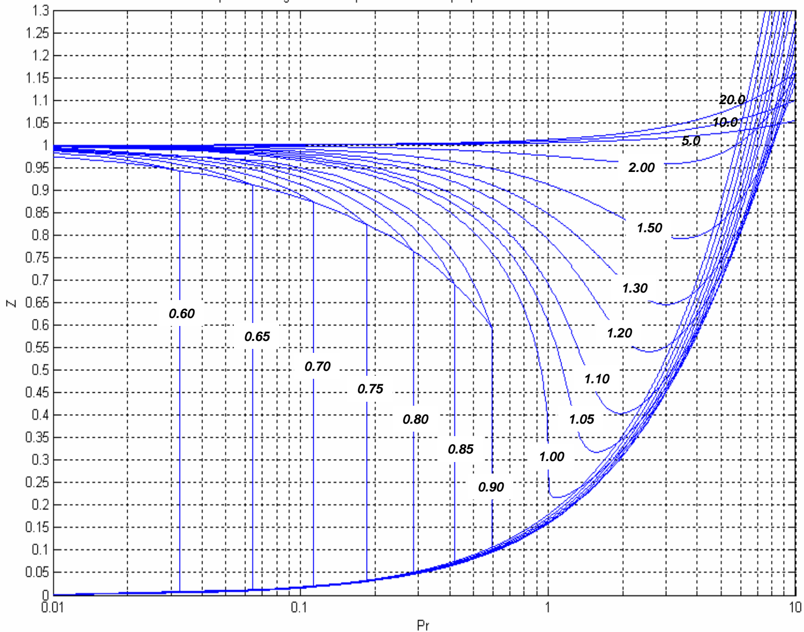
Carta de compresibilidad generalizada para un fluido simple por la ecuación de estado de Lee & Kesler
